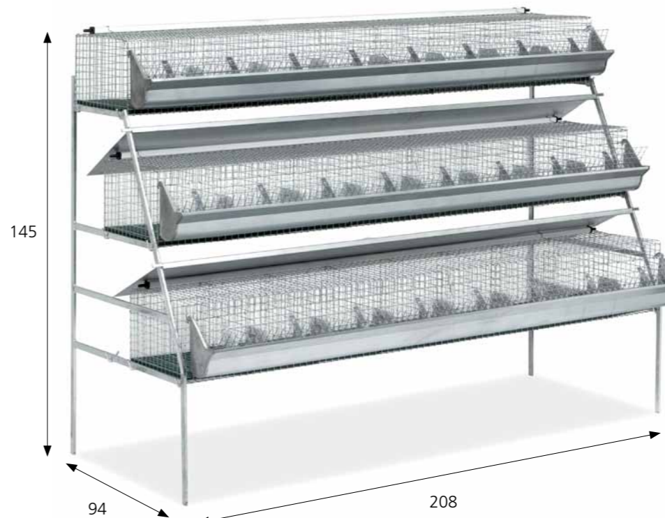
box ingrasso fattening box case engraissement | cm 25x36x26h
