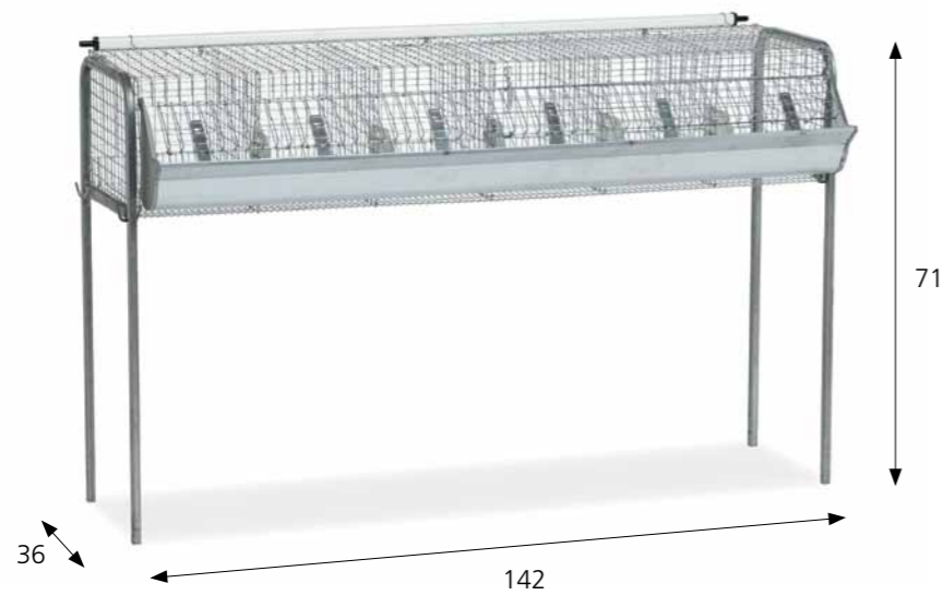
box ingrasso fattening box case engraissement | cm 25x36x26h
