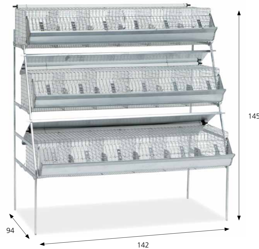
box ingrasso fattening box case engraissement | cm 25x36x26h
